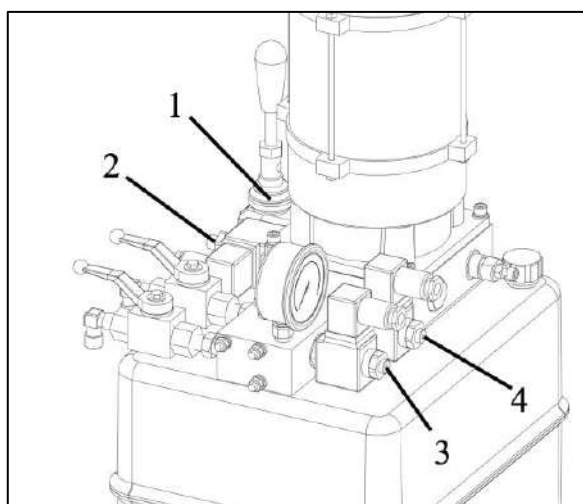
Fig. 15 - Nödsänkning av lyft och frihjulslyft
