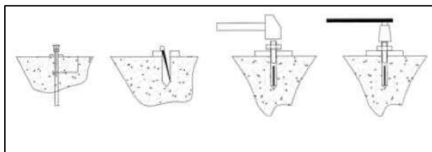
Fig. 11 - Ekspansionsboltene fastgøres i gulvet
